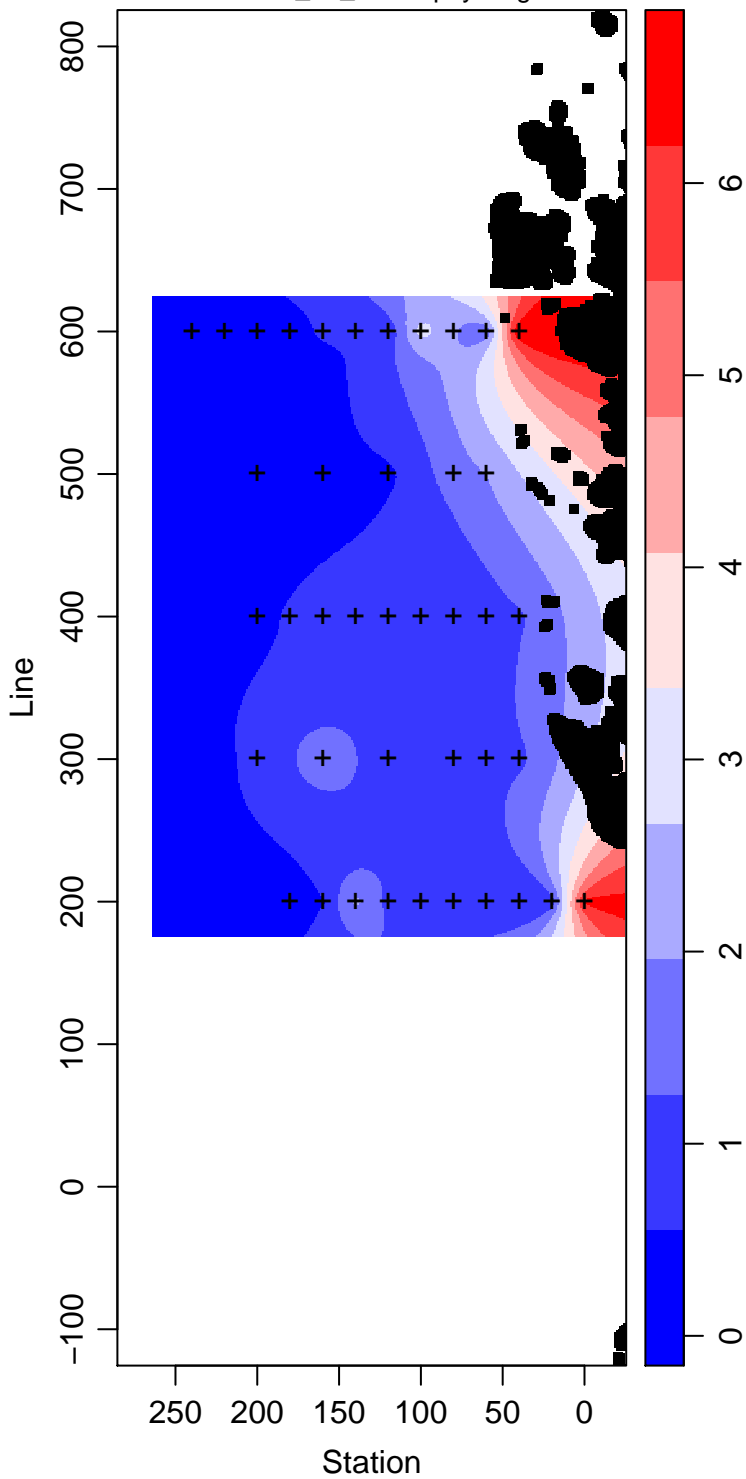
LMG00-01_10_Chlorophyll \text{mg m}^{-3}
