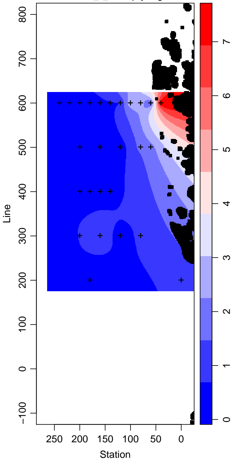
LMG00-01_1_Chlorophyll mg m -3
