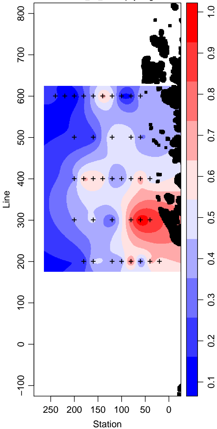
LMG00-01_35_Chlorophyll mg m -3
