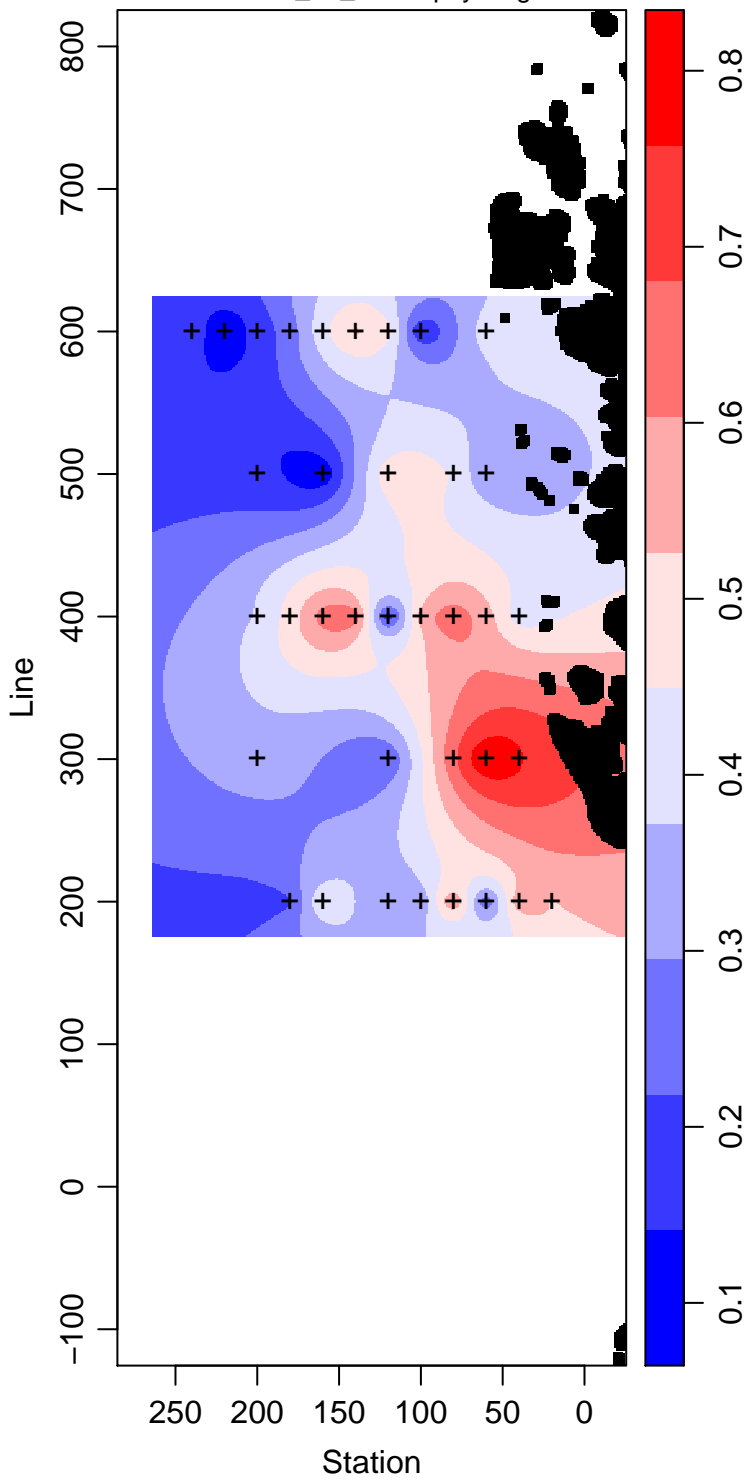
LMG00-01_40_Chlorophyll mg m -3
