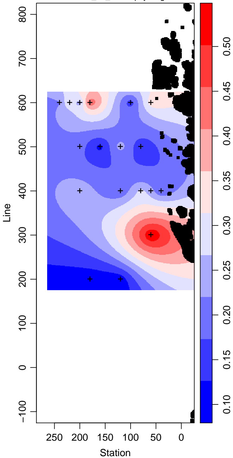
LMG00-01_65_Chlorophyll mg m -3
