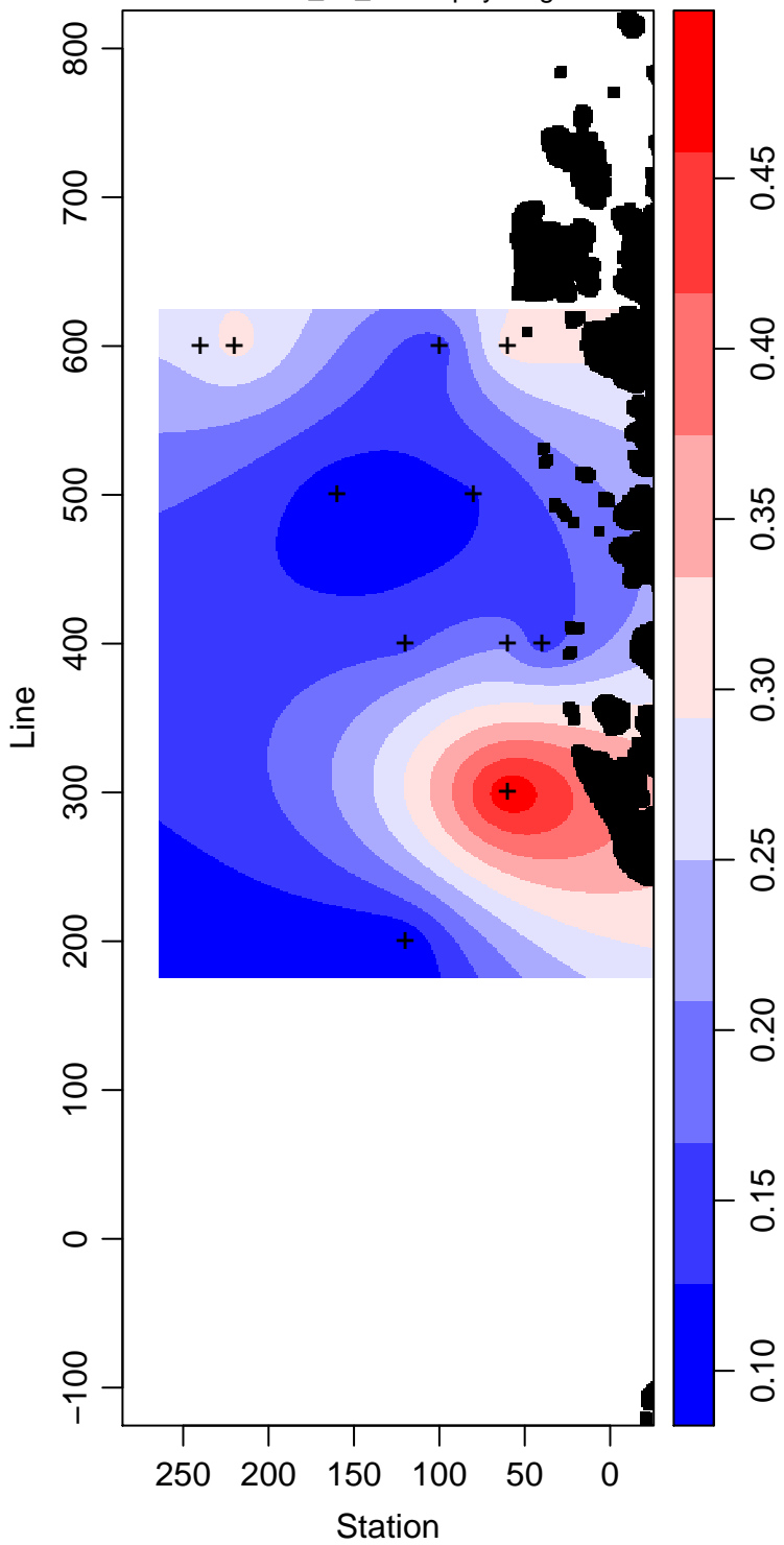
LMG00-01_75_Chlorophyll mg m -3
