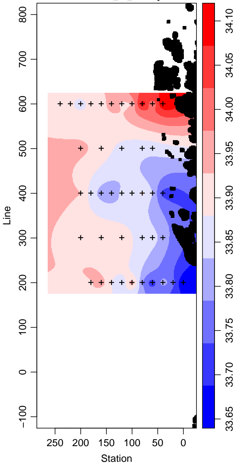
LMG00-01_50_Salinity
