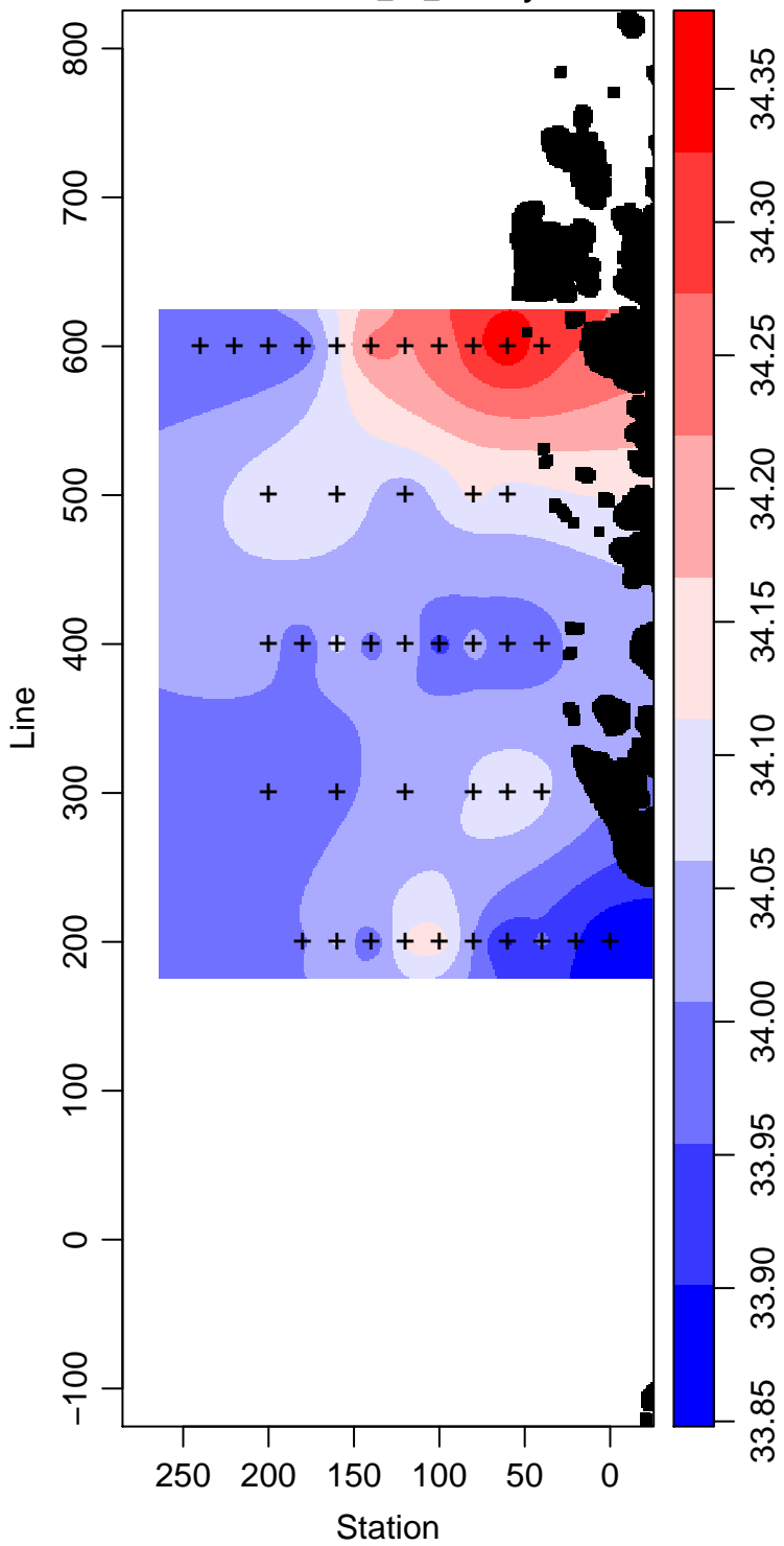
LMG00-01_75_Salinity
