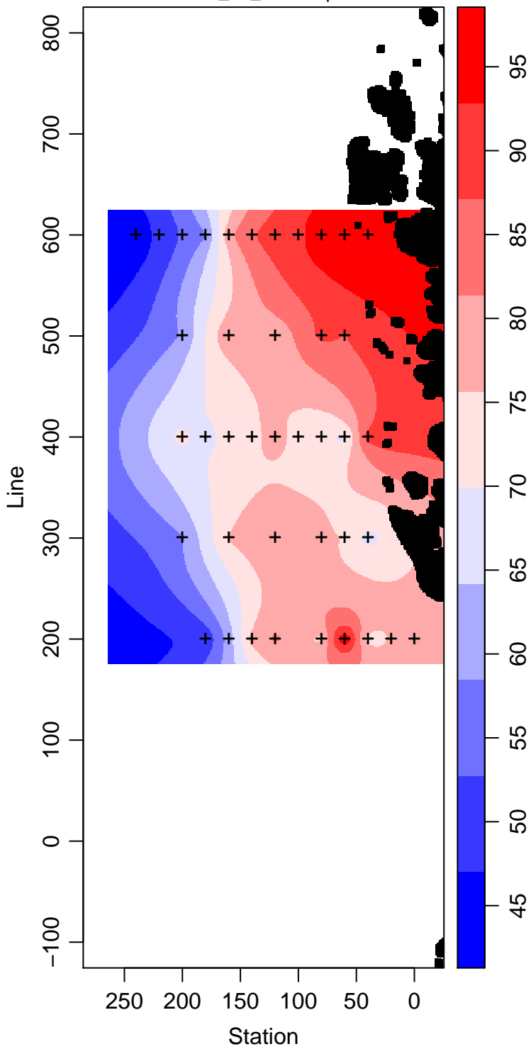
LMG00-01_70_Silicate \mu\text{ mol L}^{-1}
