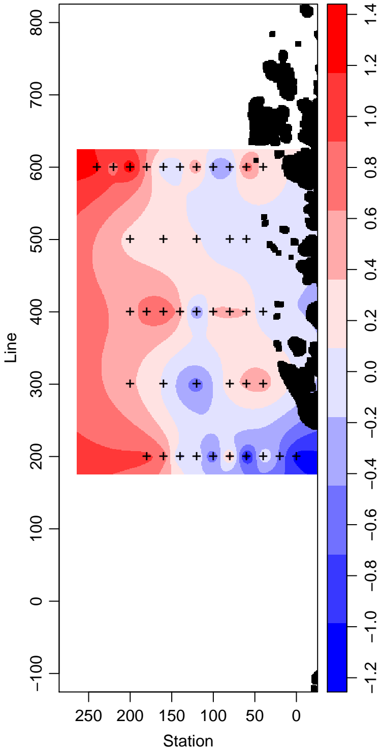
LMG00-01_40_Temperature ° Celsius
