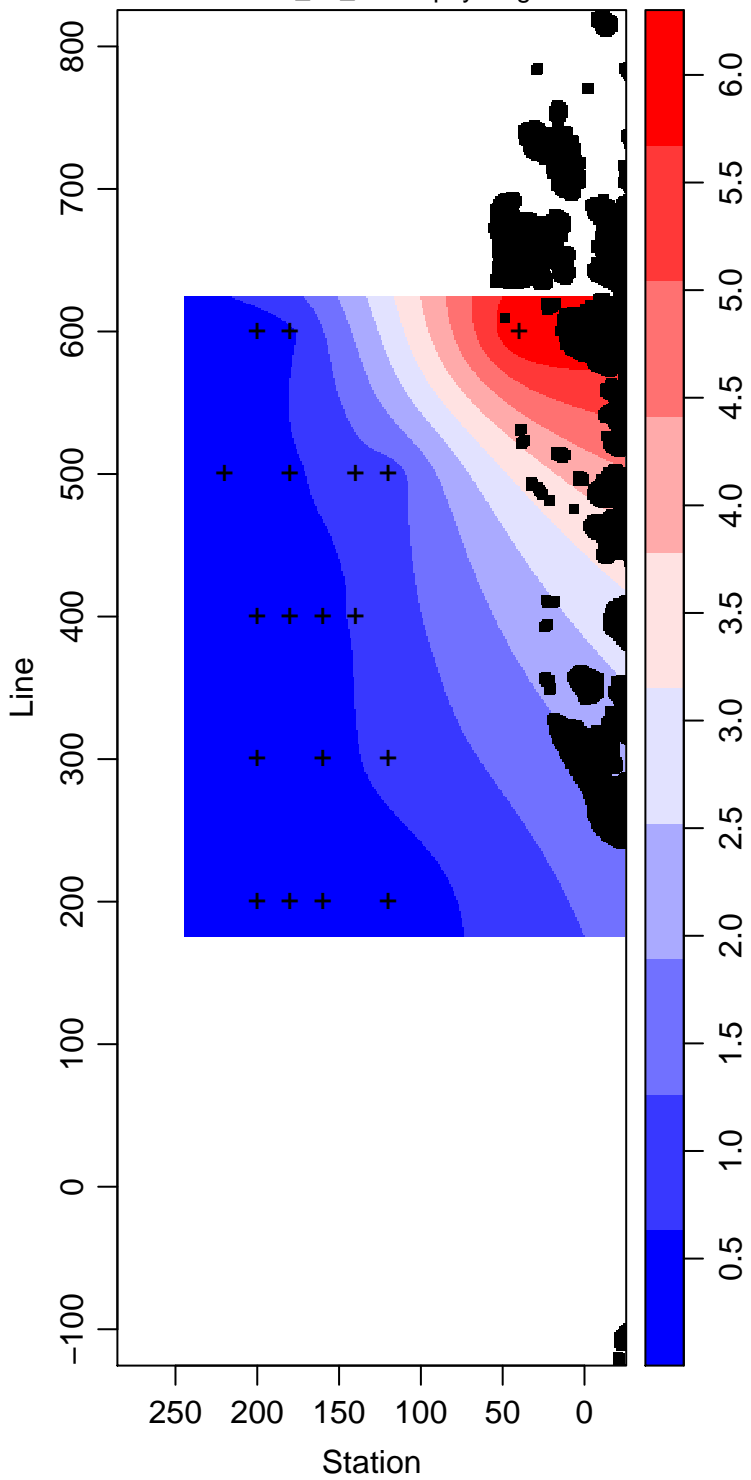
LMG01-01_45_Chlorophyll mg m -3
