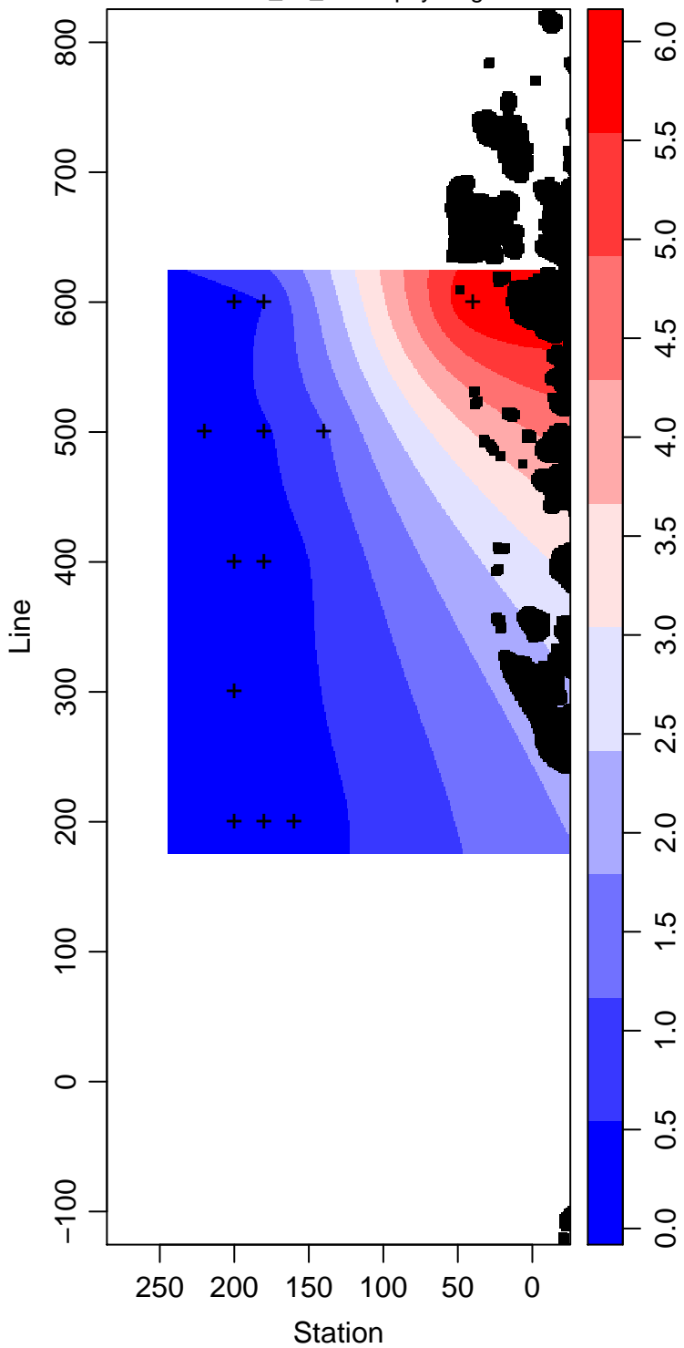
LMG01-01_55_Chlorophyll mg m -3
