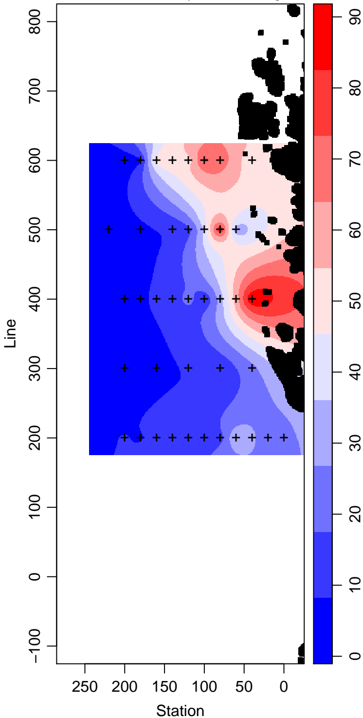
LMG01-01_10_Primary.Production mg m -3
