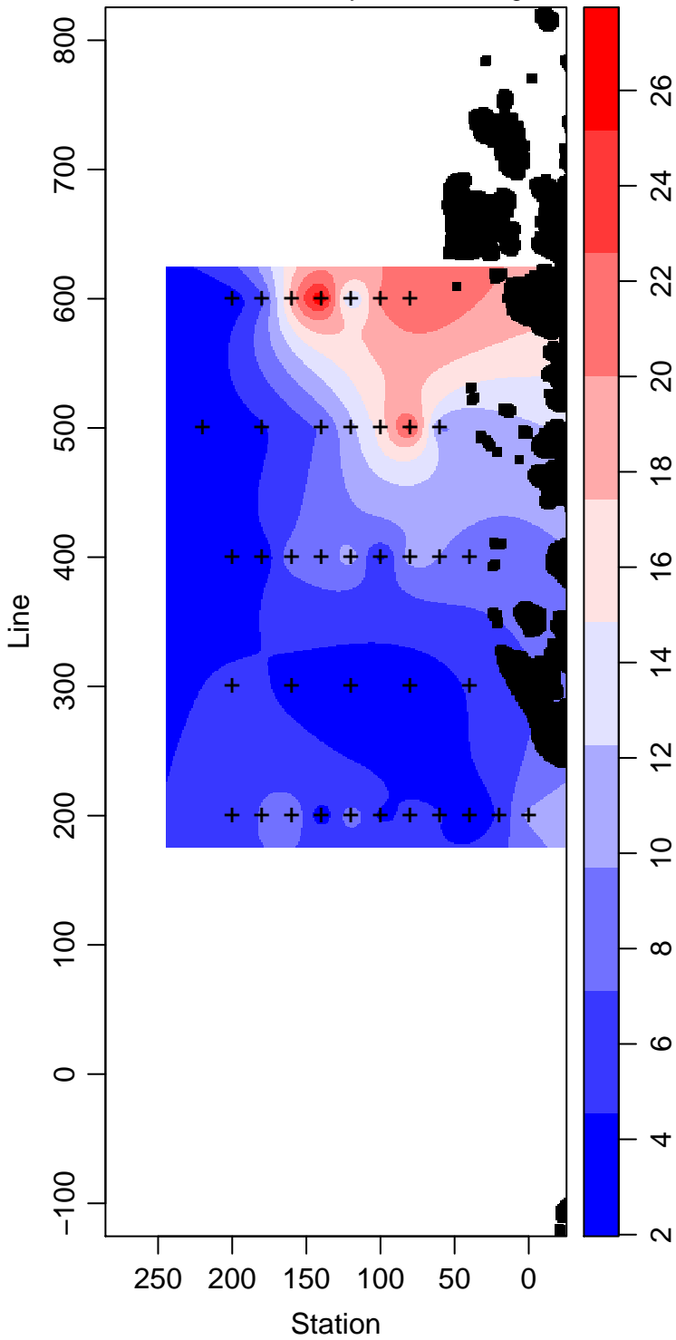
LMG01-01_25_Primary.Production mg m -3
