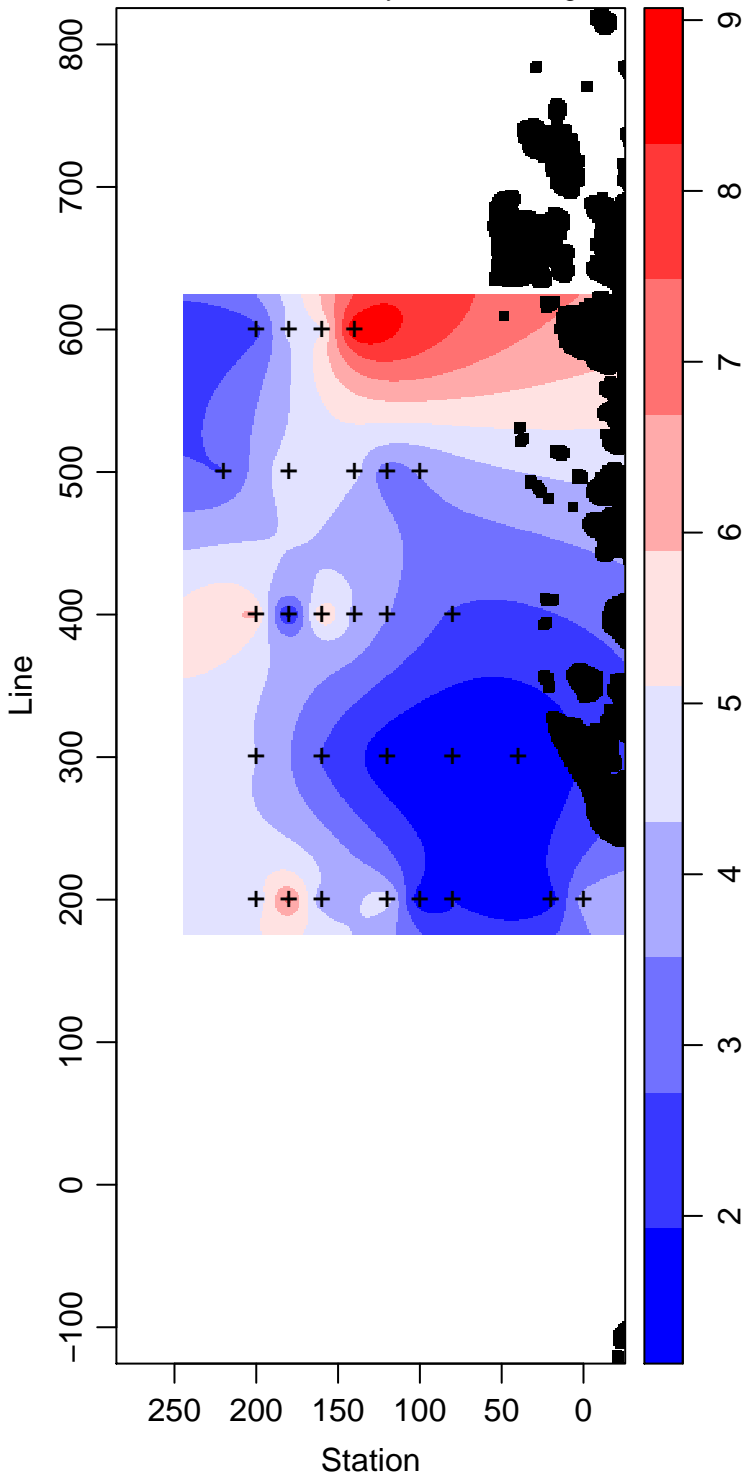
LMG01-01_35_Primary.Production mg m -3
