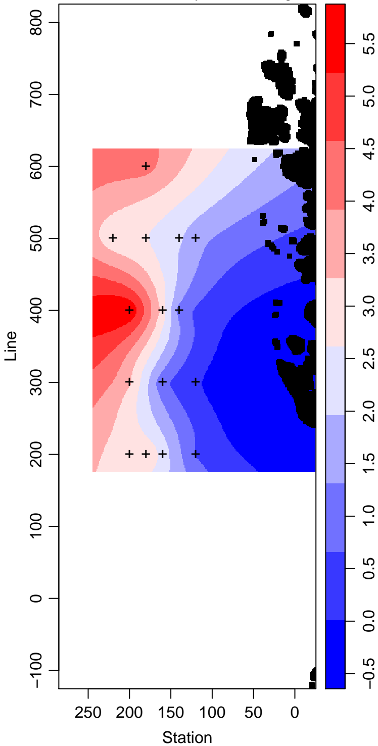
LMG01-01_45_Primary.Production mg m -3
