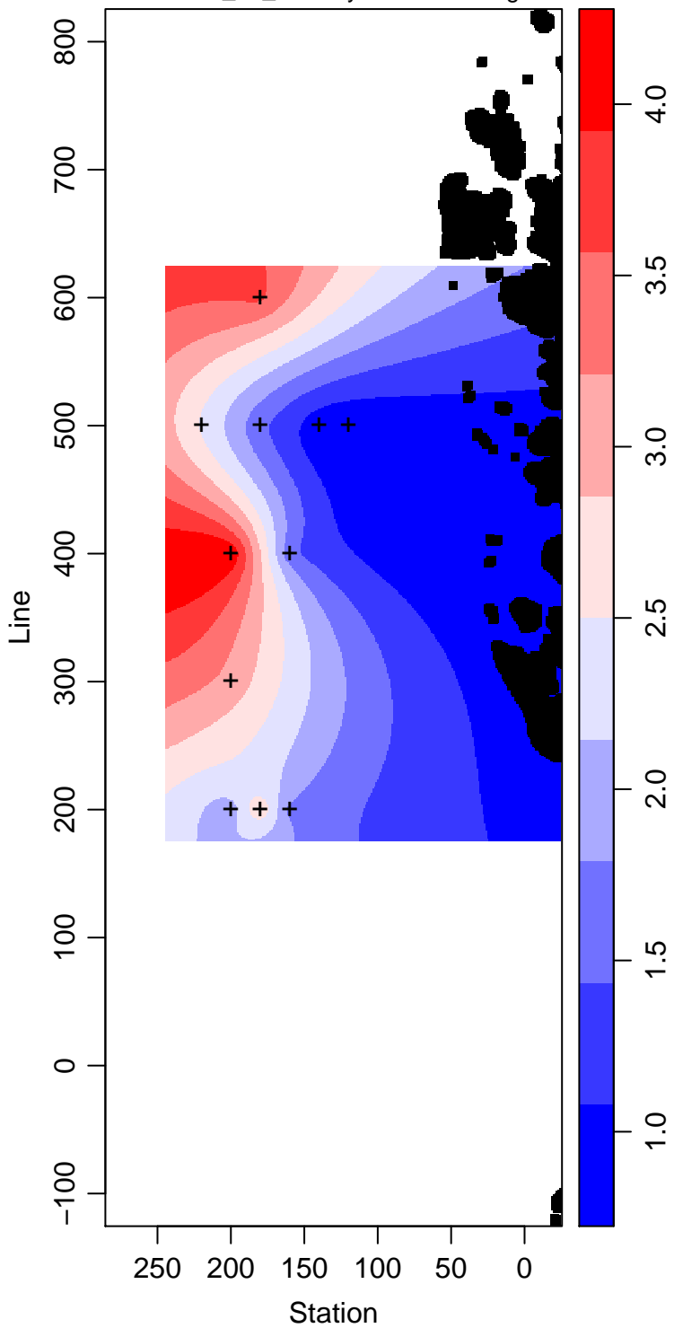
LMG01-01_50_Primary.Production mg m -3
