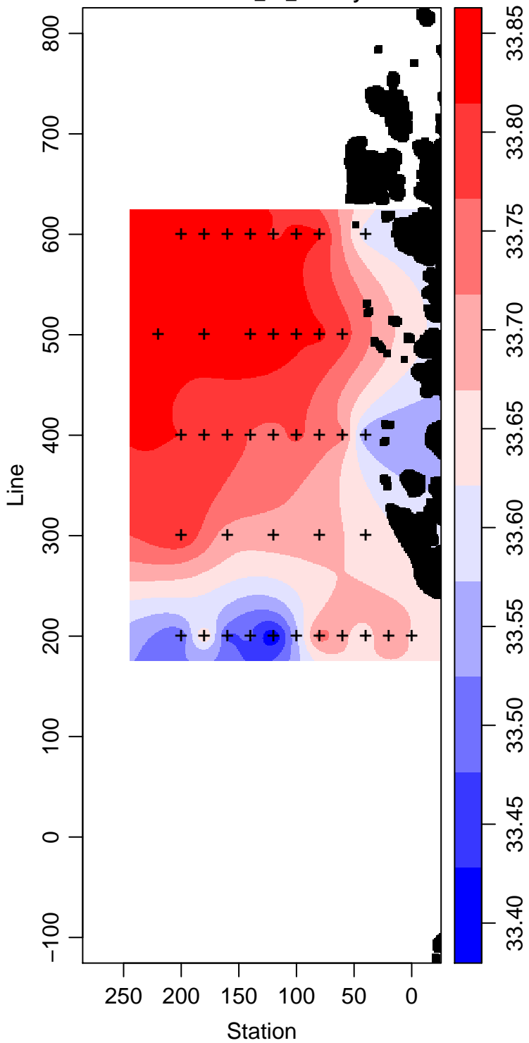
LMG01-01_10_Salinity
