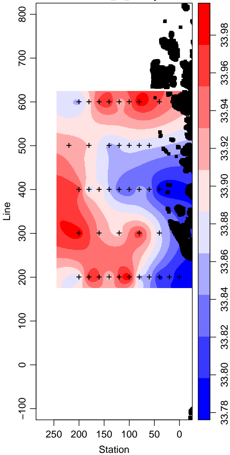
LMG01-01_50_Salinity
