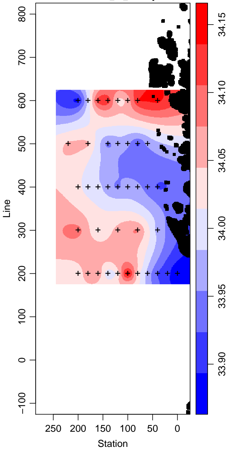
LMG01-01_70_Salinity
