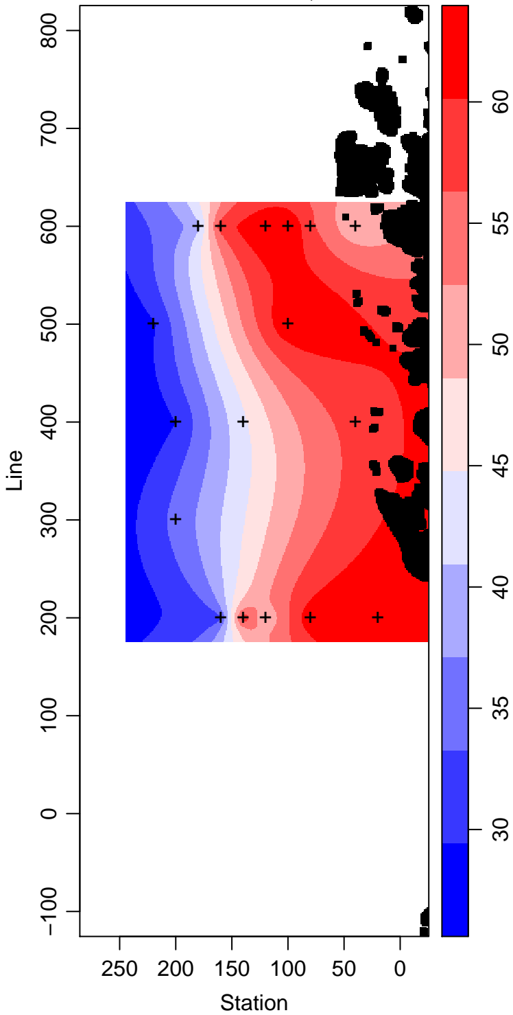
LMG01-01_1_Silicate \mu\text{ mol L}^{-1}
