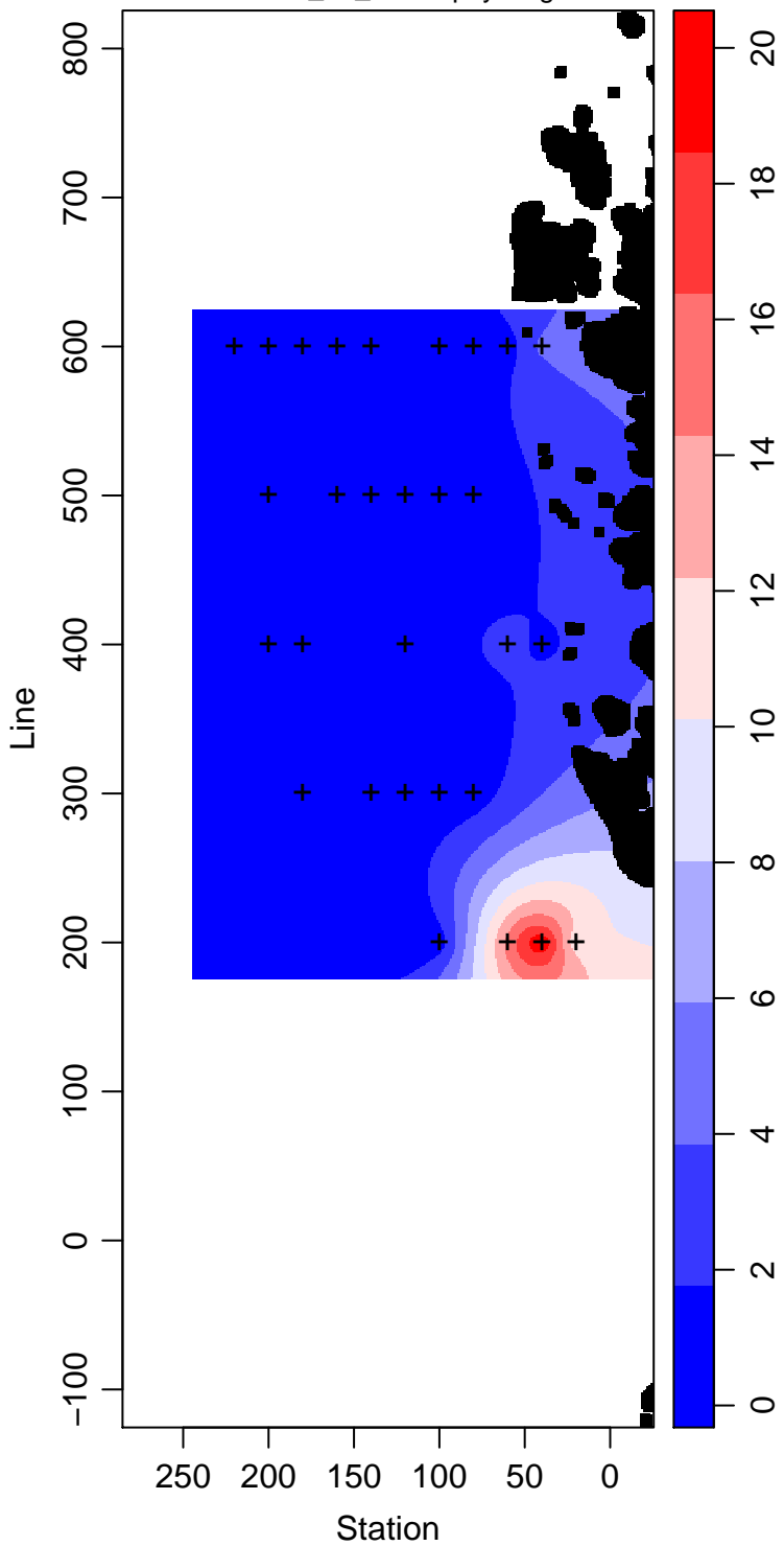
LMG02-01_10_Chlorophyll mg m -3
