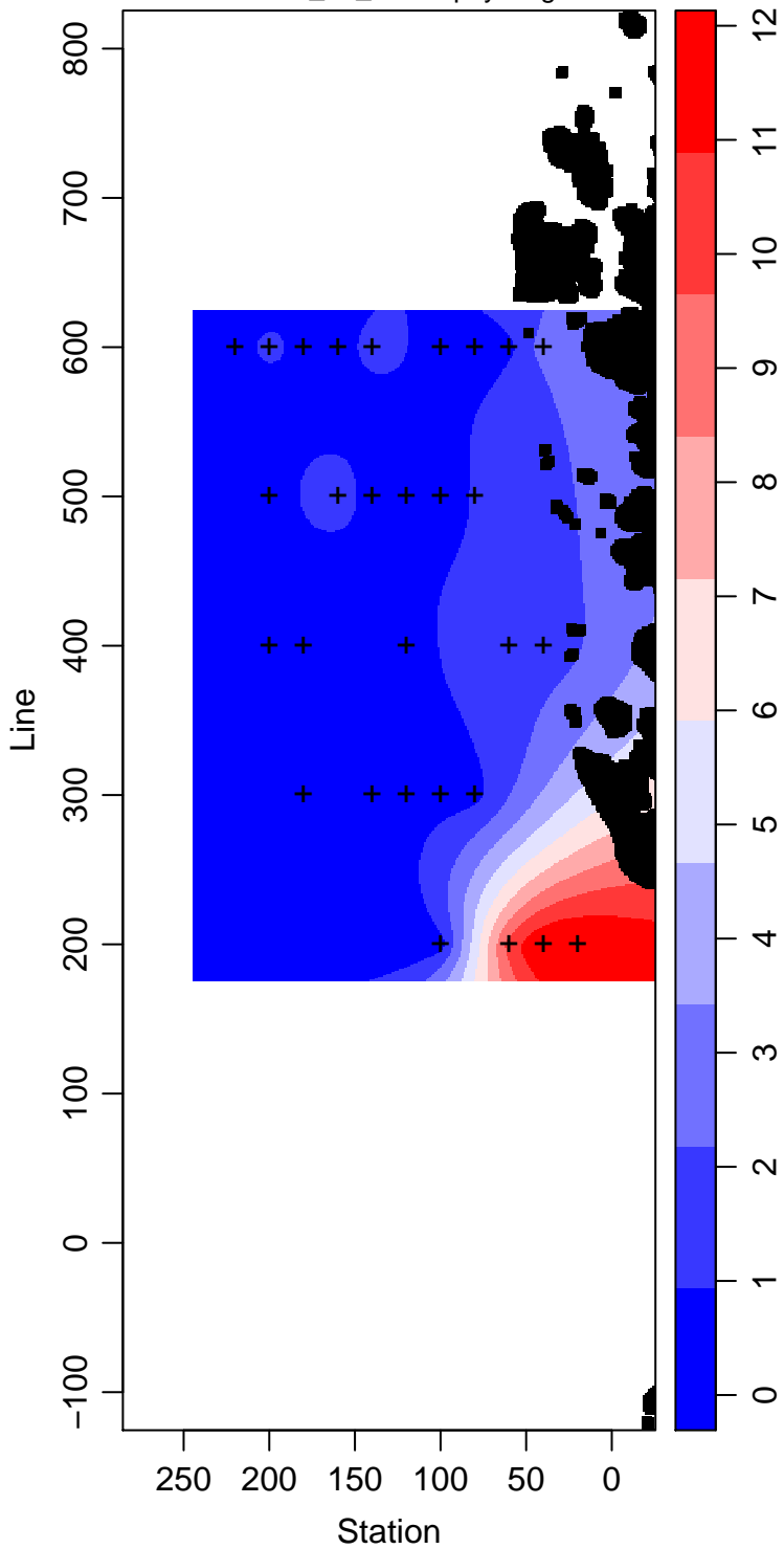
LMG02-01_30_Chlorophyll mg m -3
