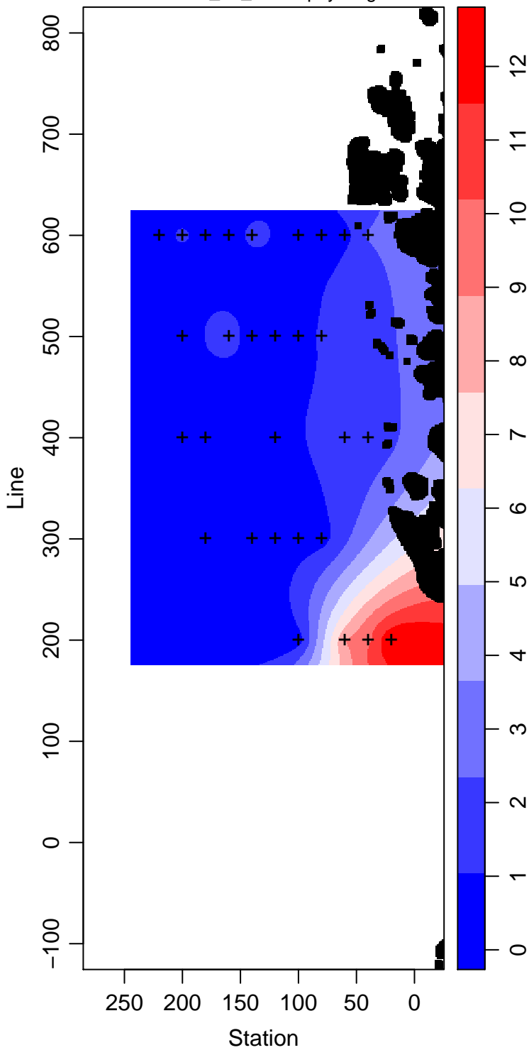
LMG02-01_35_Chlorophyll mg m -3
