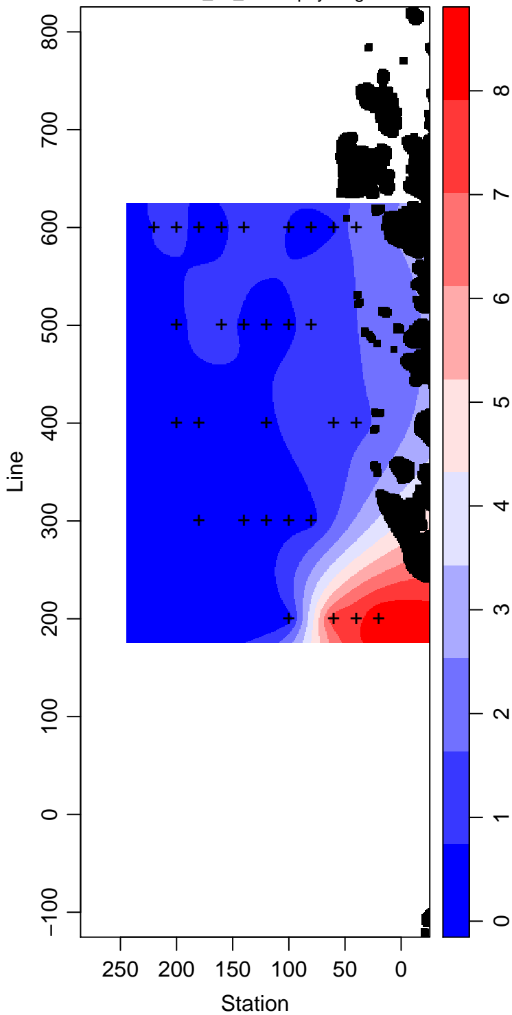
LMG02-01_40_Chlorophyll mg m -3
