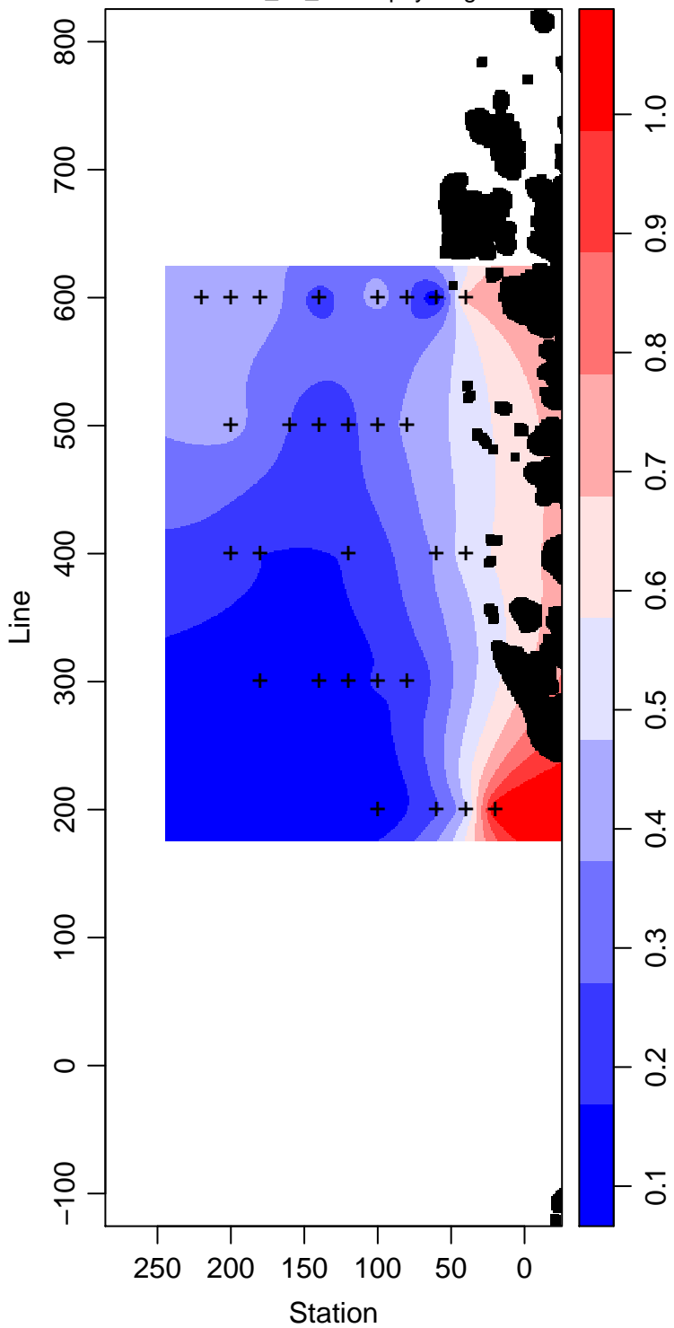
LMG02-01_80_Chlorophyll mg m -3
