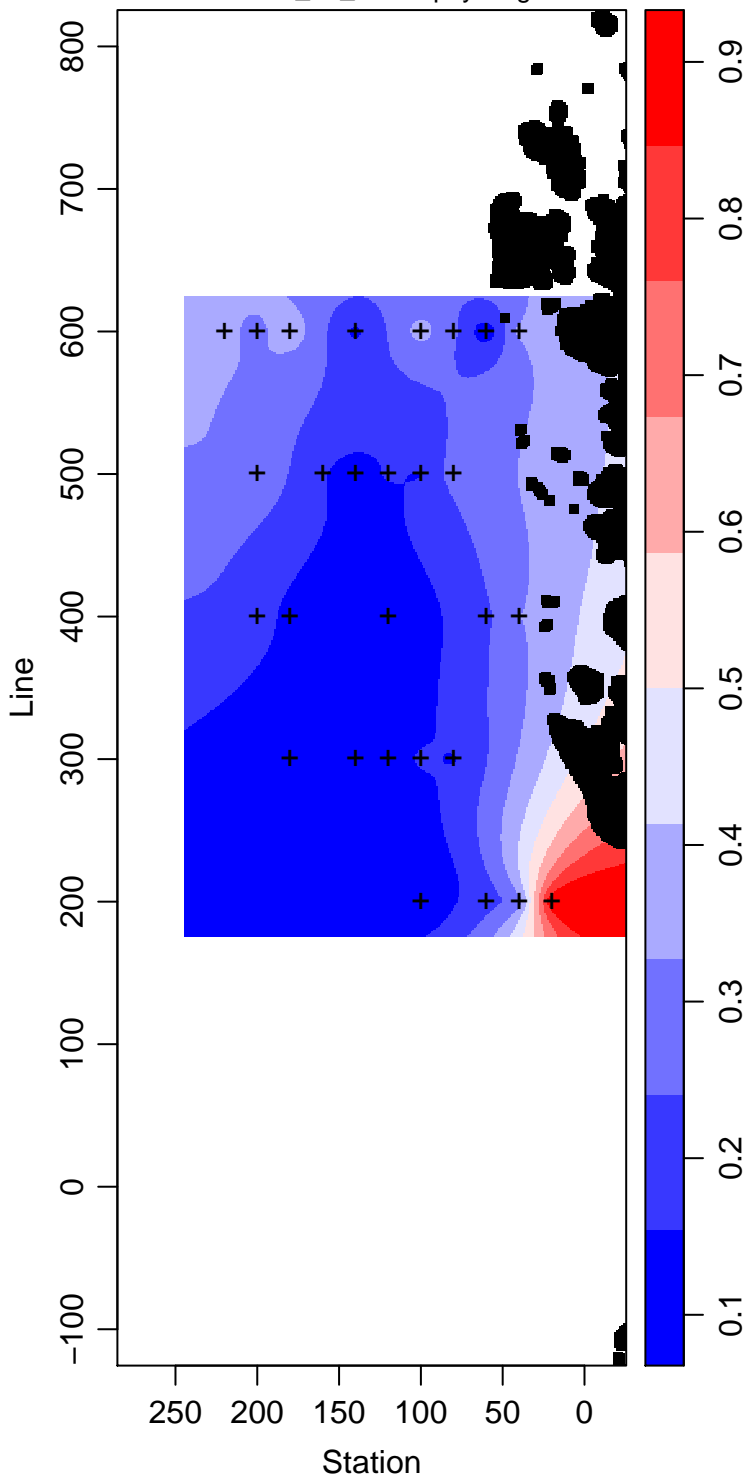
LMG02-01_90_Chlorophyll mg m -3
