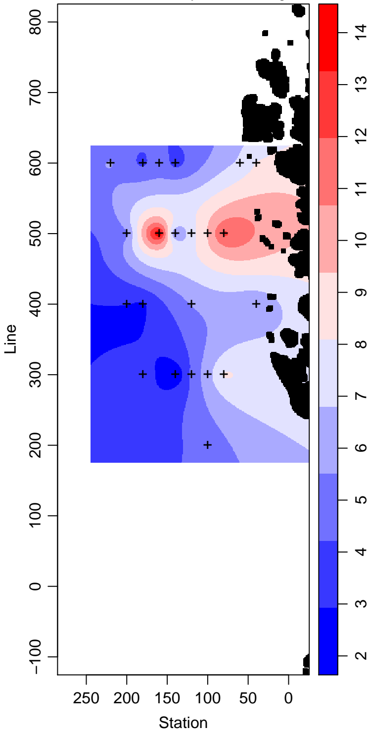
LMG02-01_35_Primary.Production mg m -3
