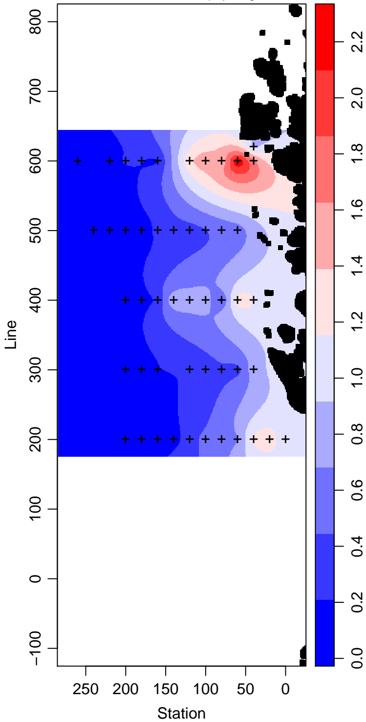
LMG03-01_1_Chlorophyll mg m -3
