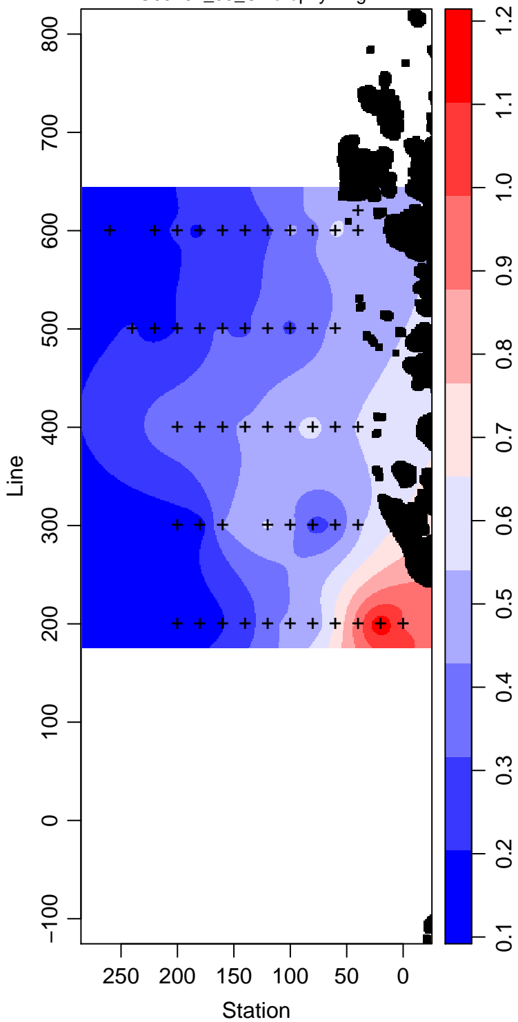
LMG03-01_35_Chlorophyll mg m -3
