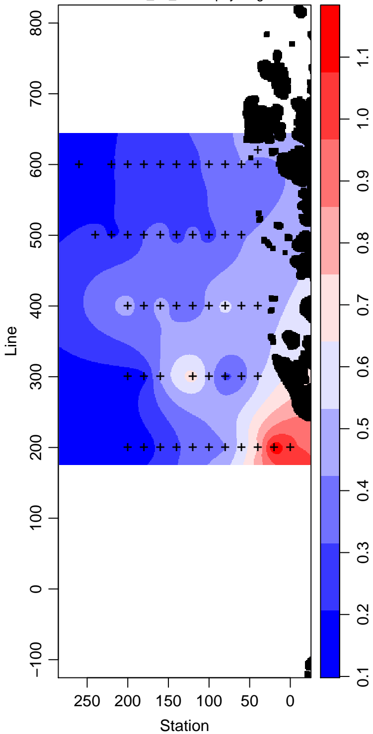
LMG03-01_40_Chlorophyll mg m -3
