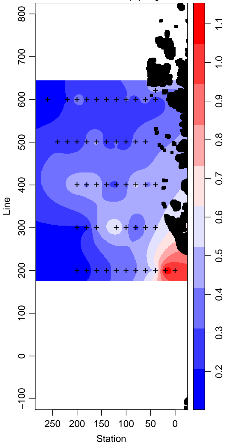
LMG03-01_45_Chlorophyll mg m -3
