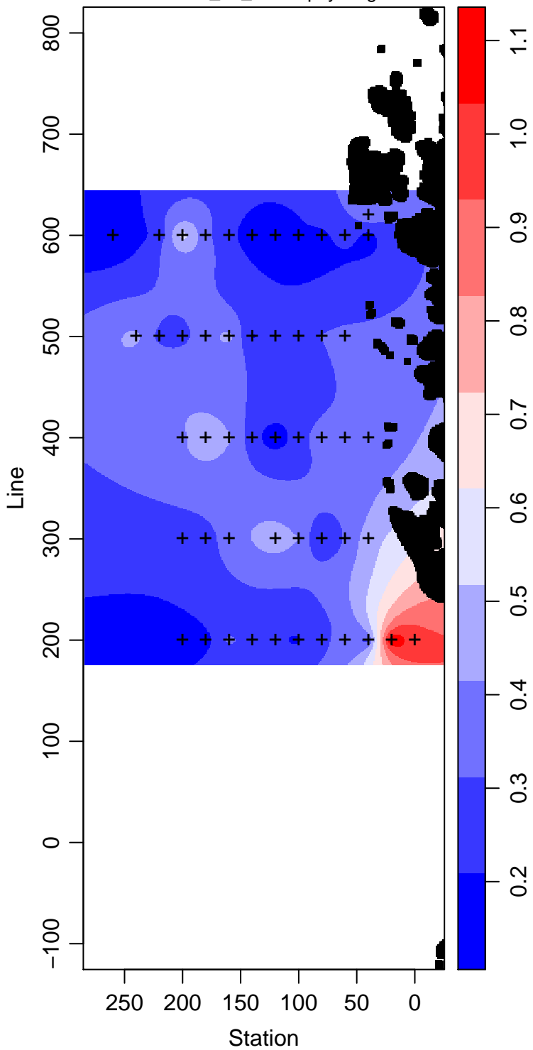
LMG03-01_55_Chlorophyll mg m -3
