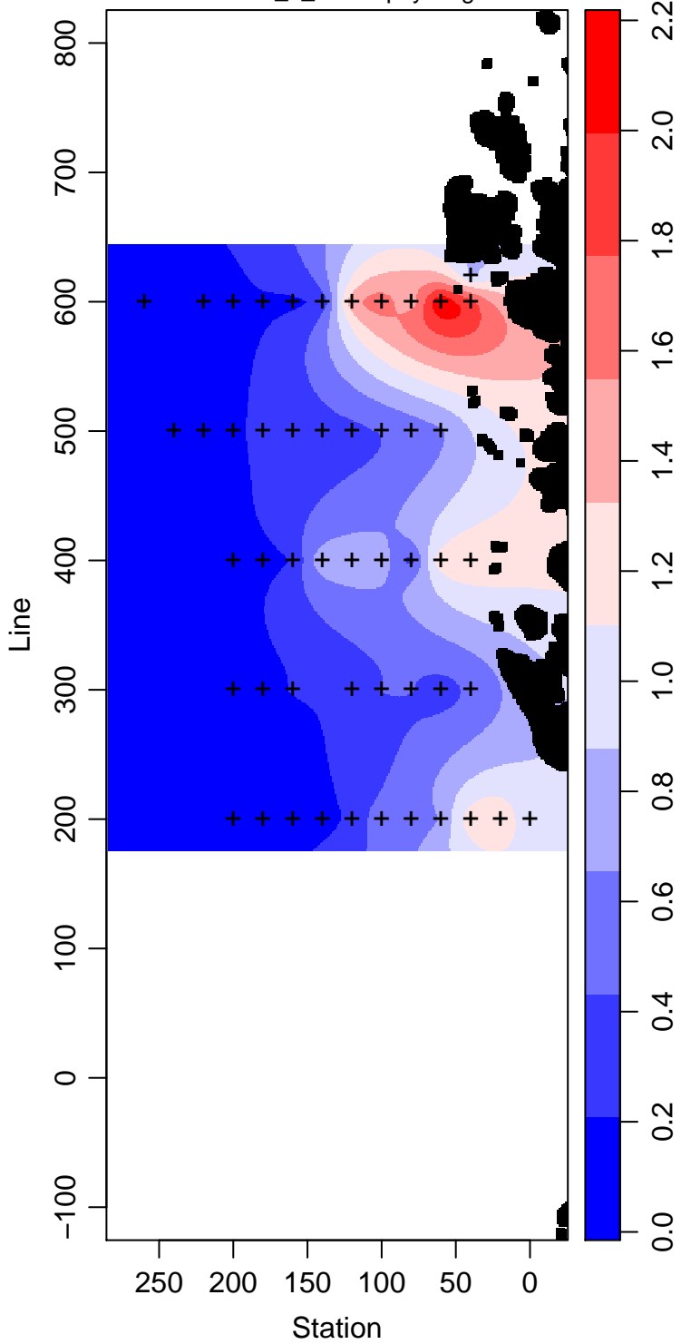
LMG03-01_5_Chlorophyll mg m -3
