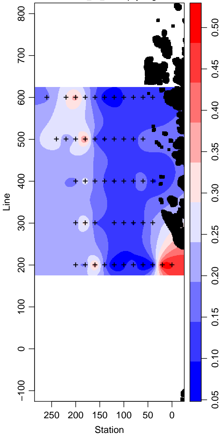
LMG03-01_80_Chlorophyll mg m -3
