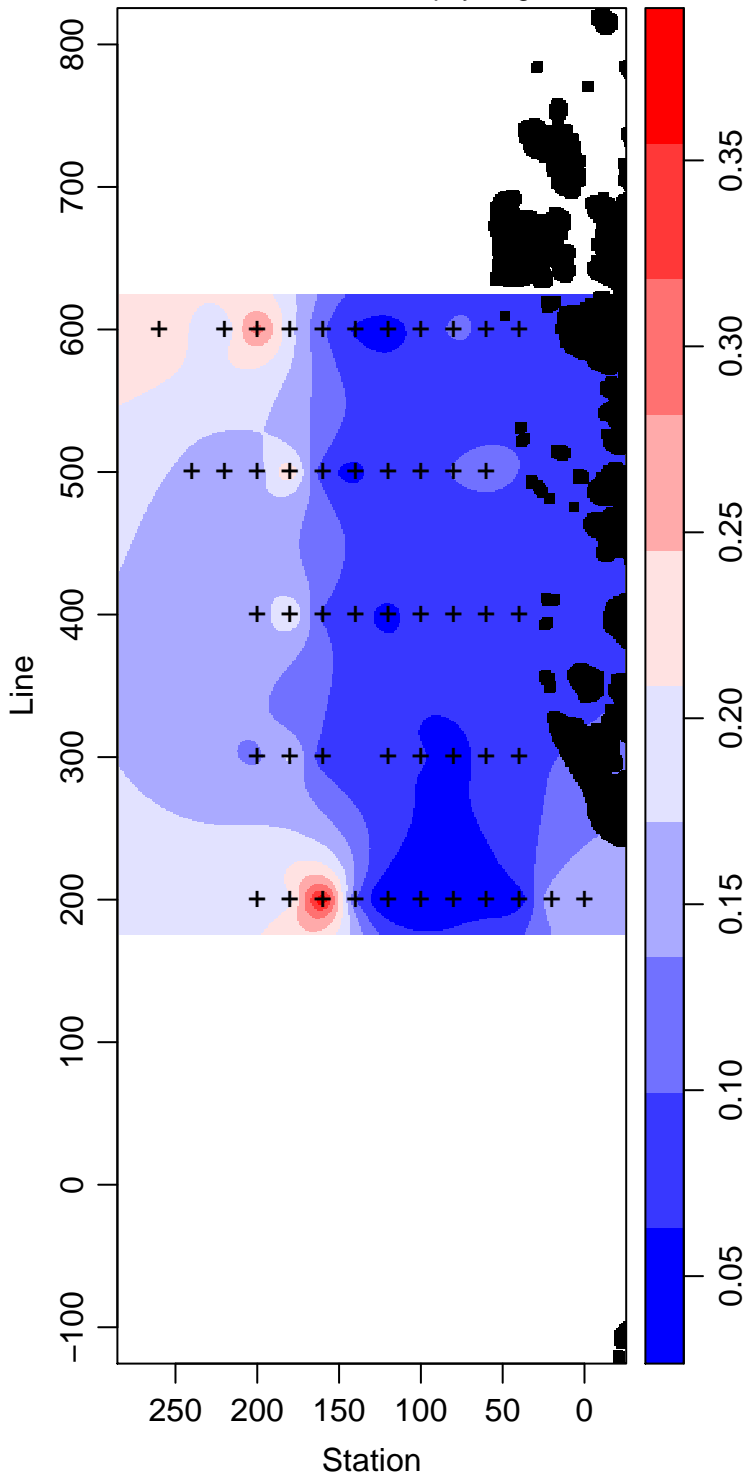
LMG03-01_95_Chlorophyll mg m -3
