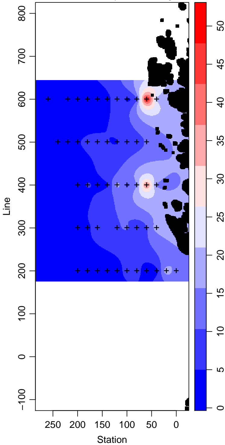
LMG03-01_1_Primary.Production mg m -3
