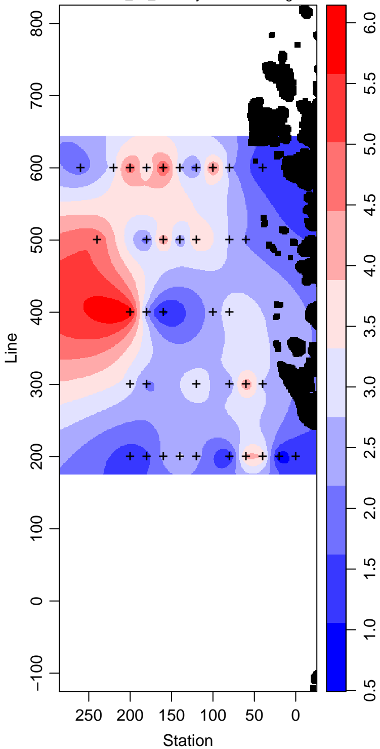
LMG03-01_55_Primary.Production mg m -3
