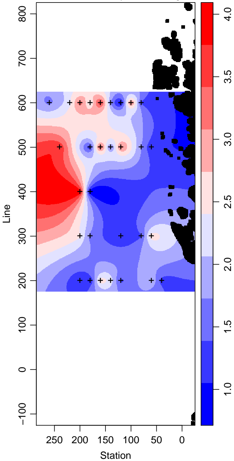
LMG03-01_65_Primary.Production mg m -3
