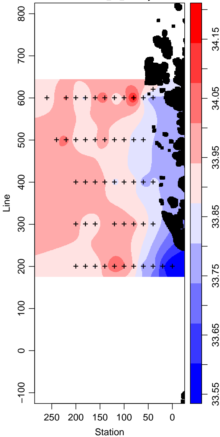
LMG03-01_60_Salinity
