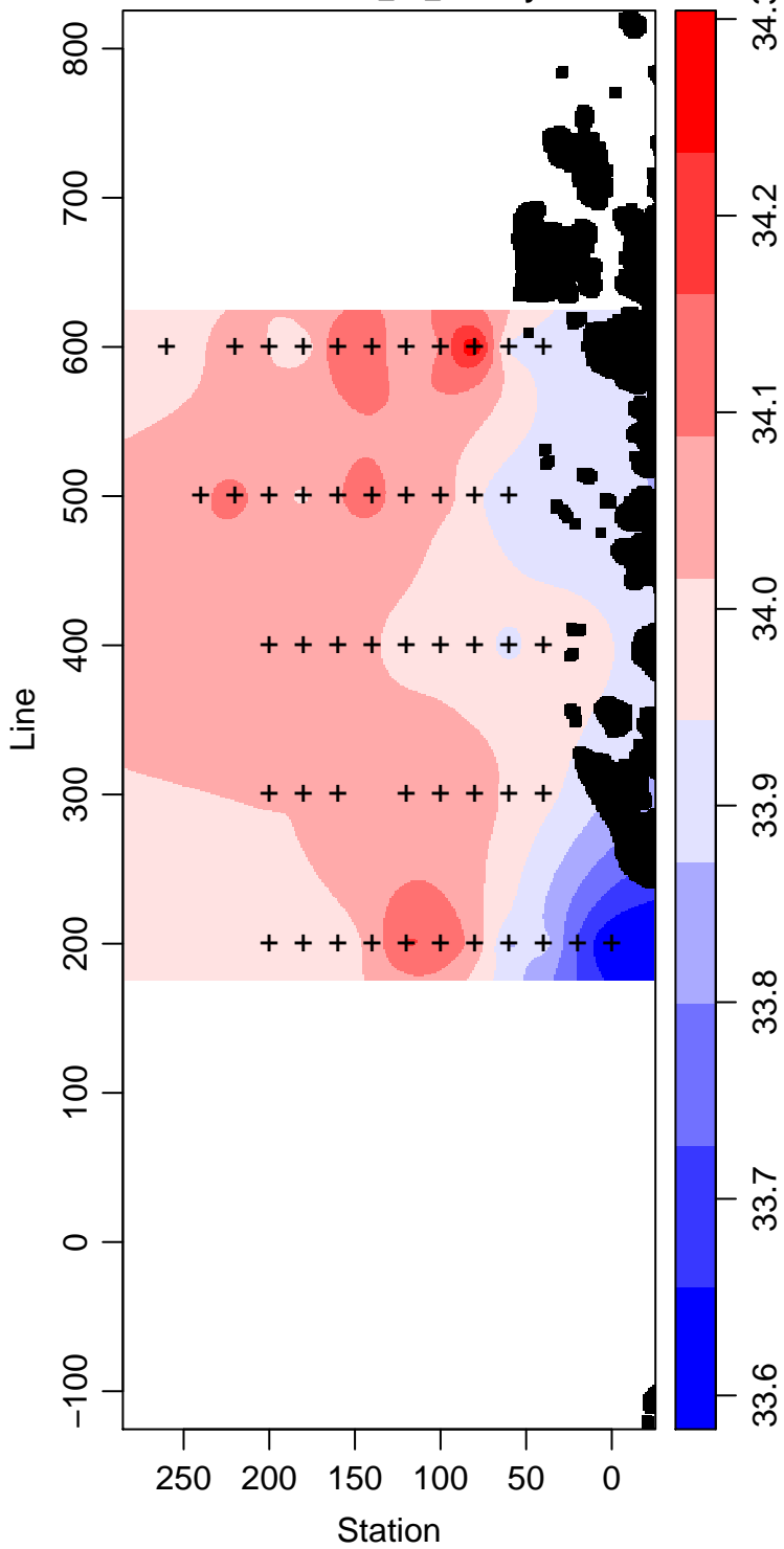
LMG03-01_75_Salinity
