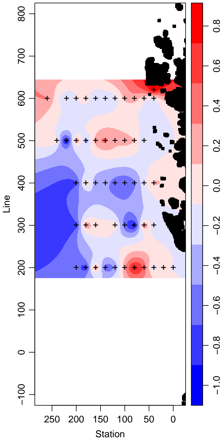
LMG03-01_40_Temperature ° Celsius
