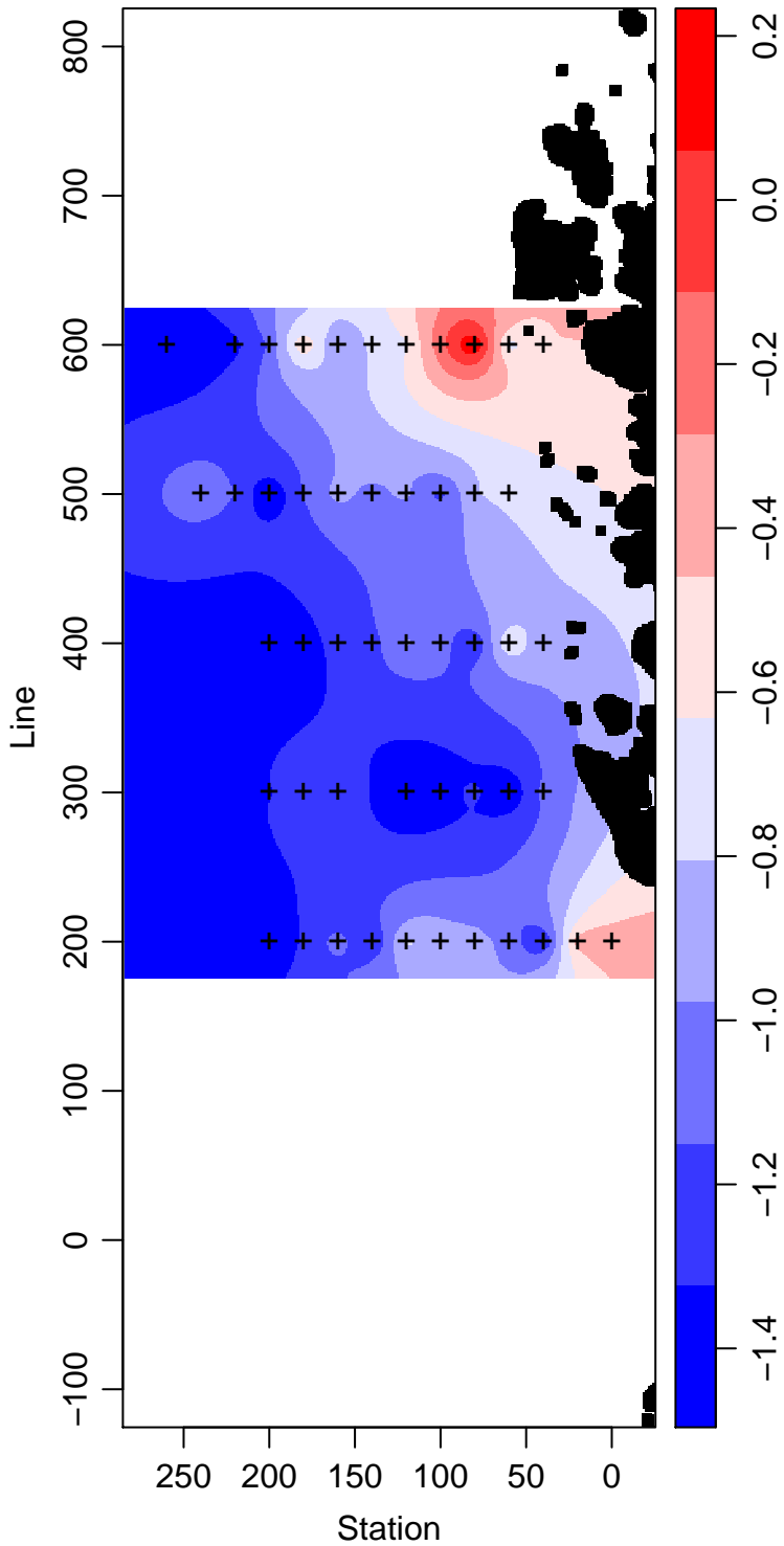
LMG03-01_70_Temperature ° Celsius
