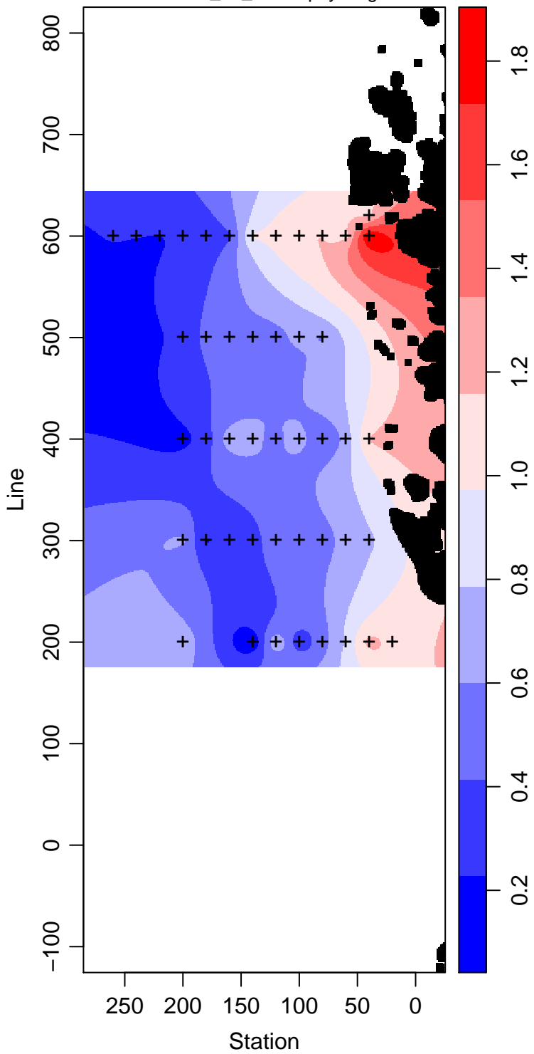
LMG04-01_15_Chlorophyll mg m -3
