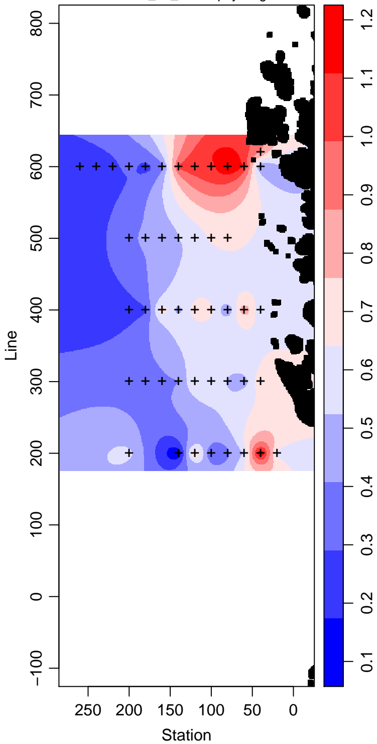
LMG04-01_30_Chlorophyll mg m -3
