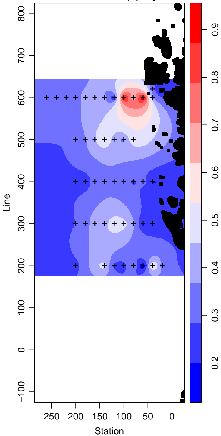
LMG04-01_60_Chlorophyll mg m -3
