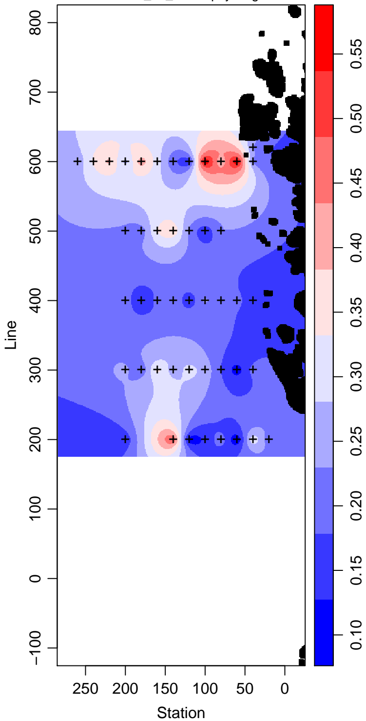
LMG04-01_80_Chlorophyll mg m -3
