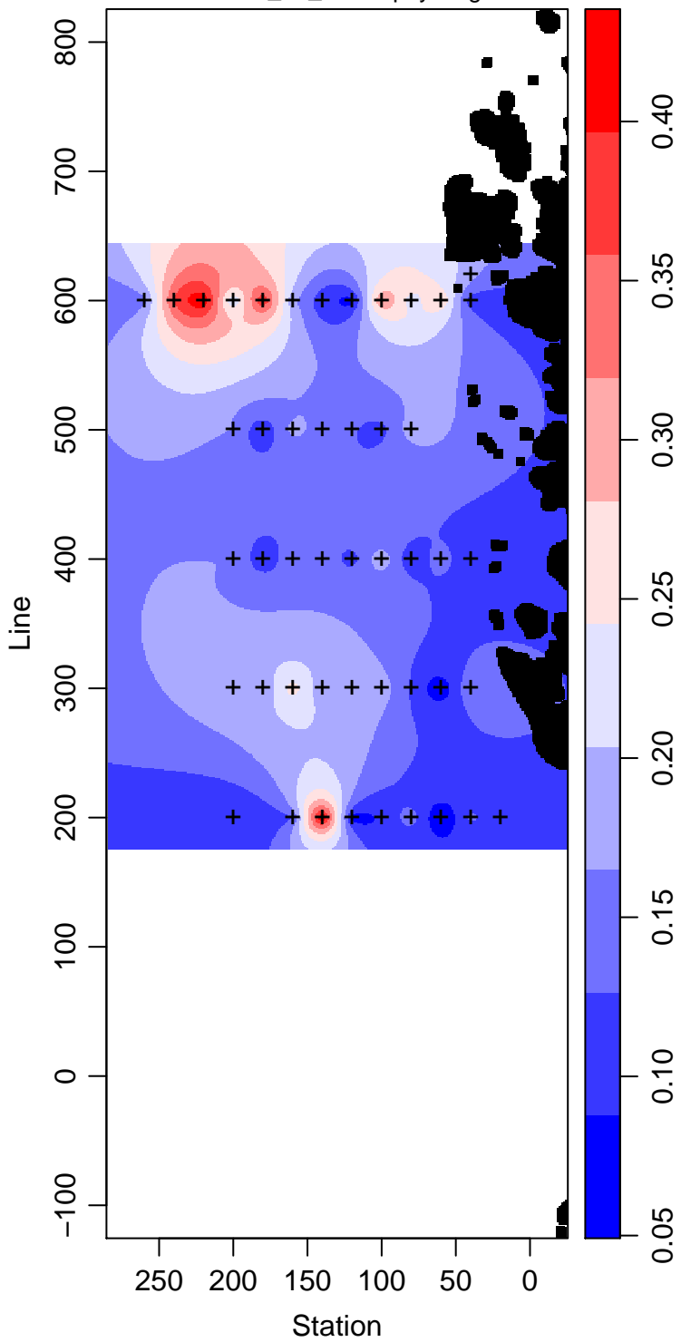
LMG04-01_95_Chlorophyll mg m -3
