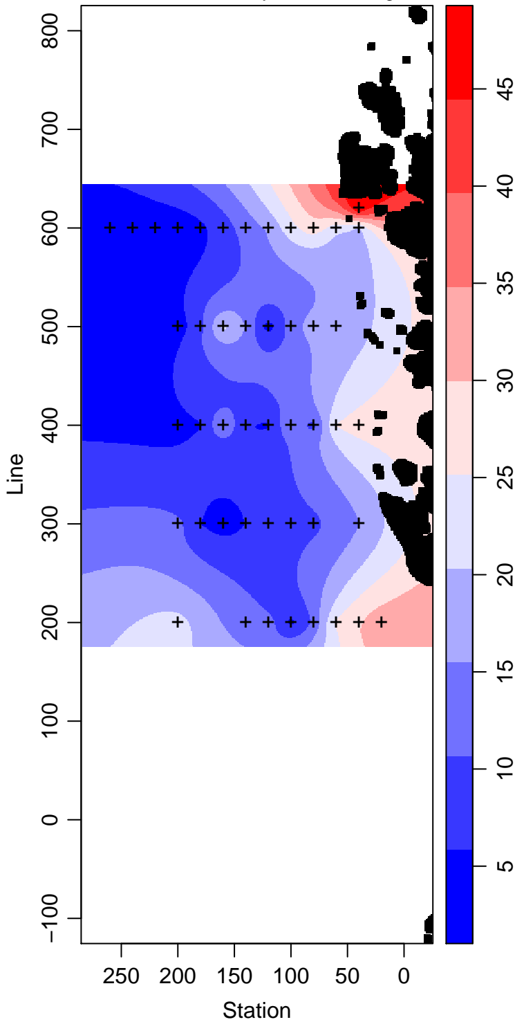
LMG04-01_5_Primary.Production mg m -3
