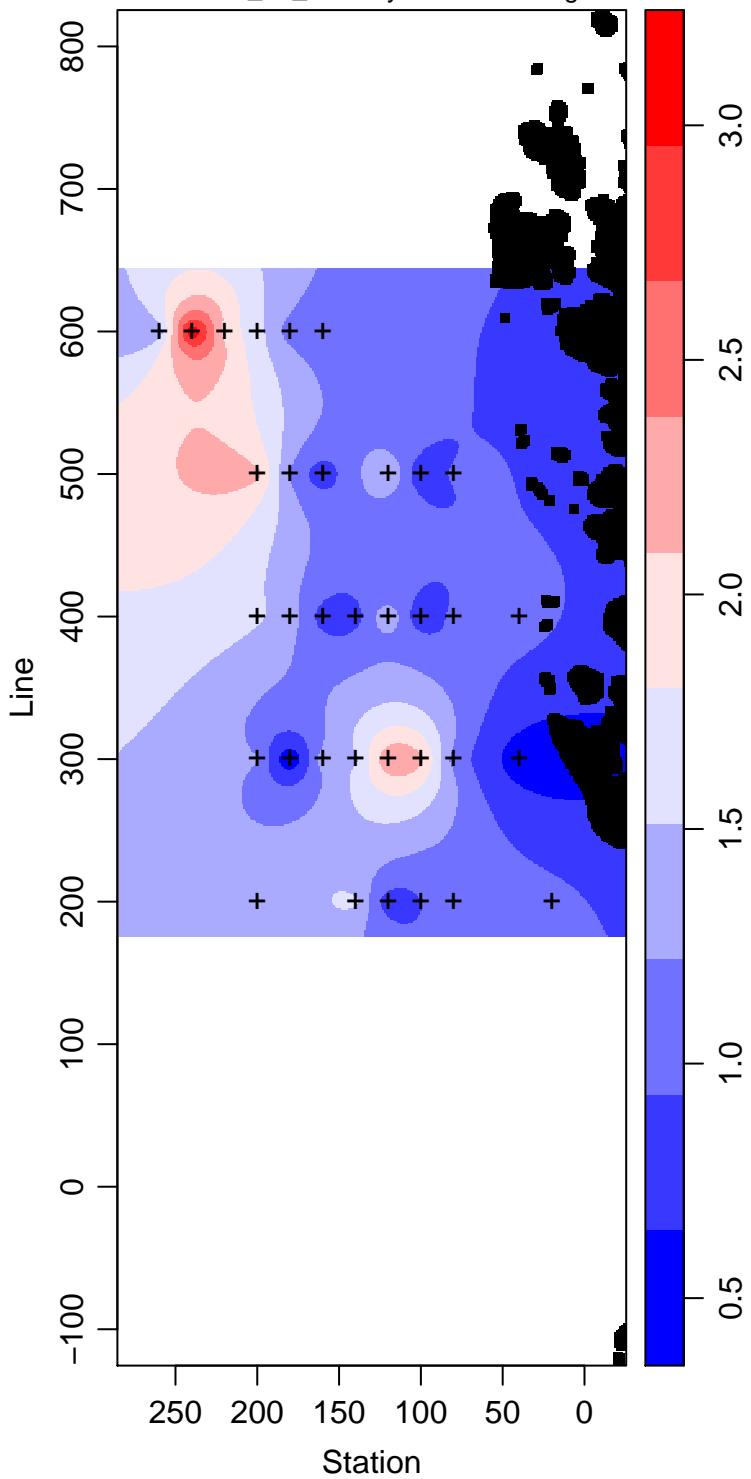
LMG04-01_70_Primary.Production mg m -3
